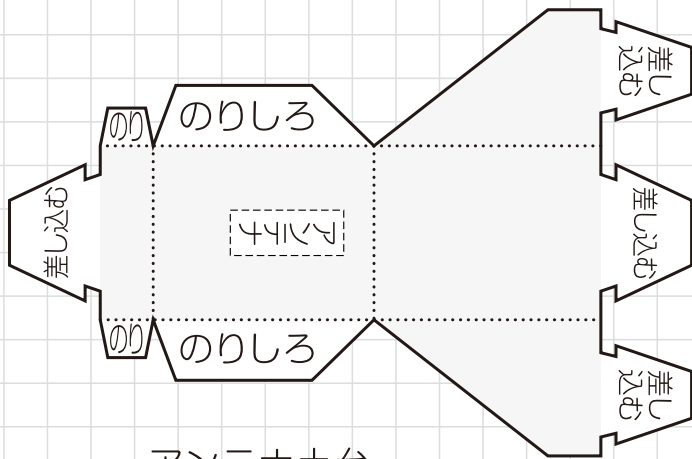
アンテナ土台
